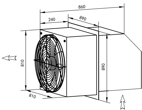
边墙送风机 WEXR-S650
