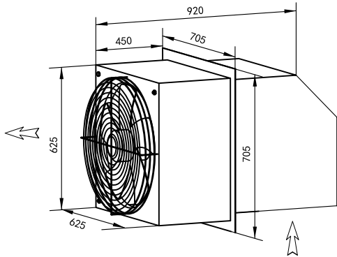
边墙送风机 WEXR-SL550
