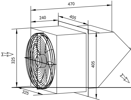
边墙排风机 WEXR-P250
