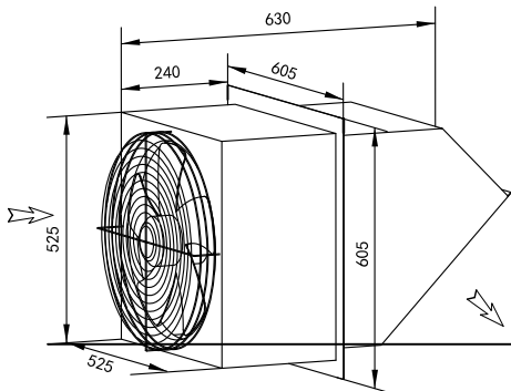
边墙排风机 WEXR-P450
