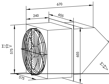
边墙排风机 WEXR-P500
