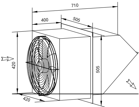
边墙排风机 WEXR-PL350
