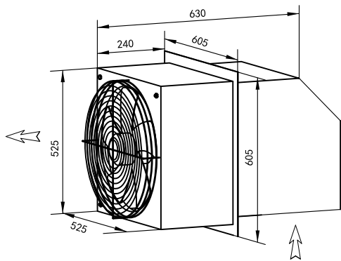
边墙送风机 WEXR-S450
