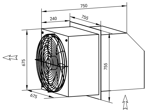
边墙送风机 WEXR-S600
