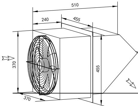
边墙排风机 WEXR-P300
