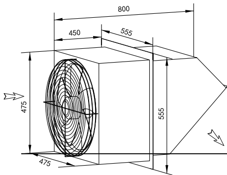
边墙排风机 WEXR-PL400
