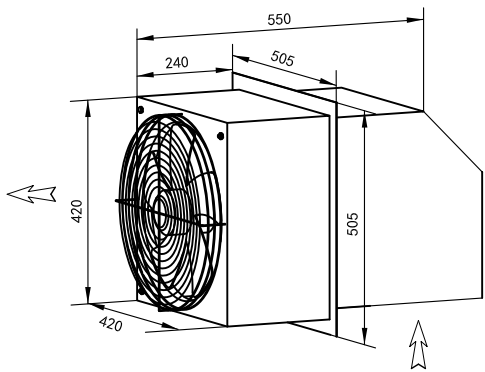
边墙送风机 WEXR-S350
