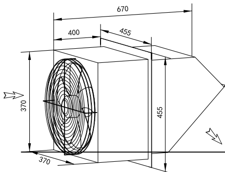
边墙排风机 WEXR-PL300
