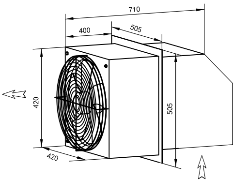
边墙送风机 WEXR-SL350
