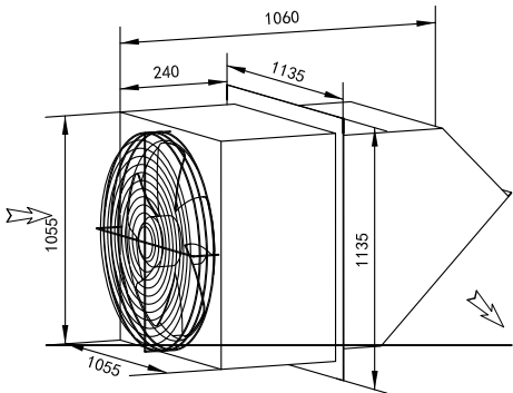
边墙排风机 WEXR-P800
