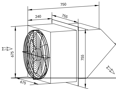
边墙排风机 WEXR-P600
