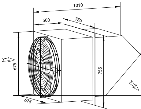
边墙排风机 WEXR-PL600
