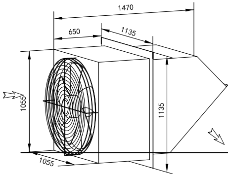
边墙排风机 WEXR-PL800
