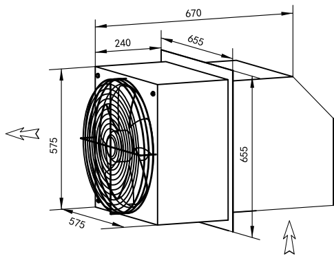
边墙送风机 WEXR-S500
