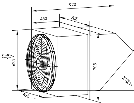
边墙排风机 WEXR-PL550
