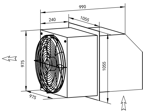
边墙送风机 WEXR-S750
