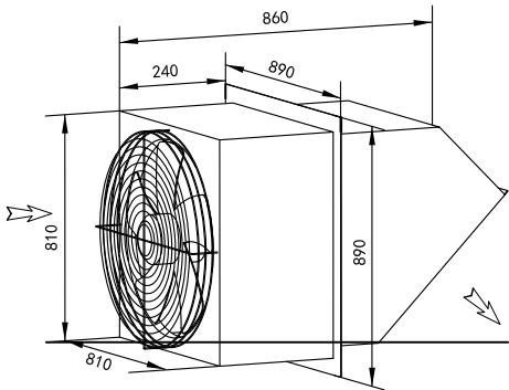
边墙排风机 WEXR-P650
