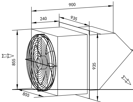
边墙排风机 WEXR-P700
