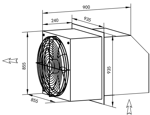
边墙送风机 WEXR-S700
