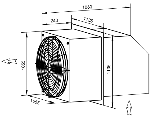
边墙送风机 WEXR-S800
