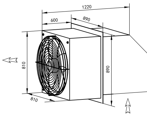
边墙送风机 WEXR-SL650
