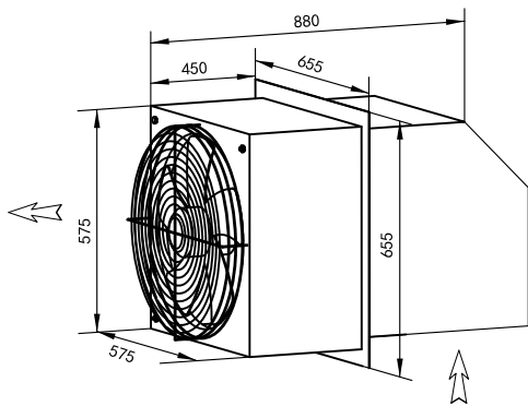
边墙送风机 WEXR-SL500
