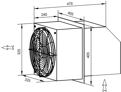
边墙送风机 WEXR-S250
