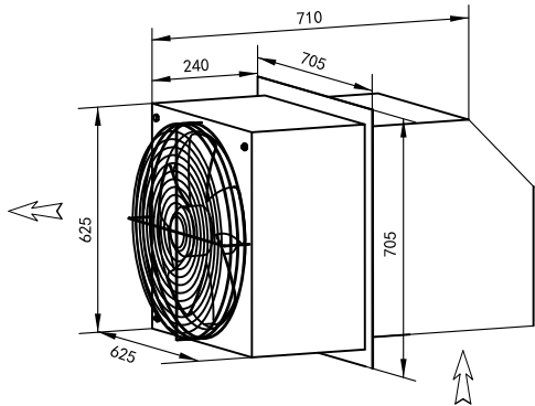
边墙送风机 WEXR-S550
