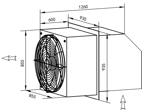
边墙送风机 WEXR-SL700
