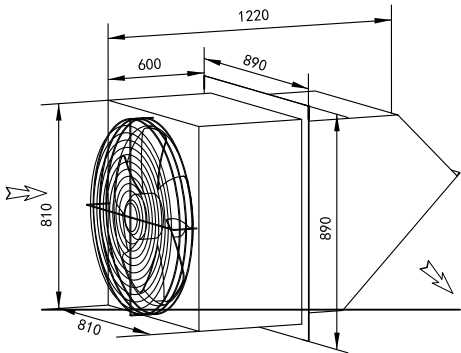
边墙排风机 WEXR-PL650
