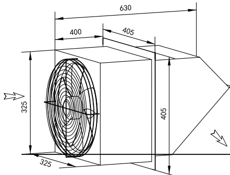
边墙排风机 WEXR-PL250
