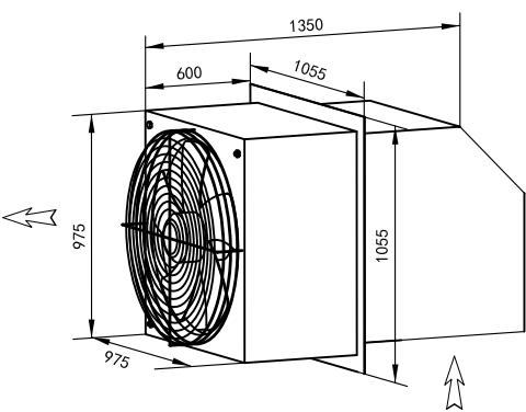
边墙送风机 WEXR-SL750
