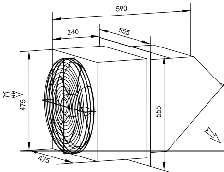
边墙排风机 WEXR-P400
