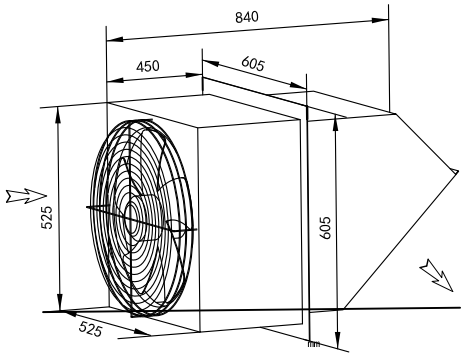
边墙排风机 WEXR-PL450
