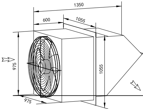
边墙排风机 WEXR-PL750
