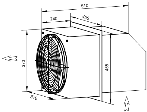
边墙送风机 WEXR-S300
