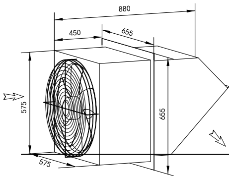
边墙排风机 WEXR-PL500
