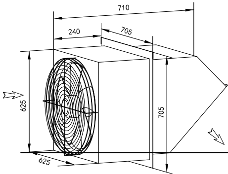
边墙排风机 WEXR-P550
