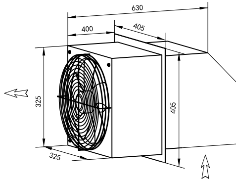
边墙送风机 WEXR-SL250
