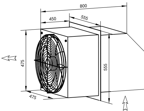
边墙送风机 WEXR-SL400
