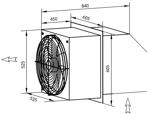
边墙送风机 WEXR-SL450
