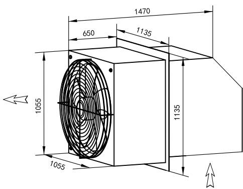
边墙送风机 WEXR-SL800
