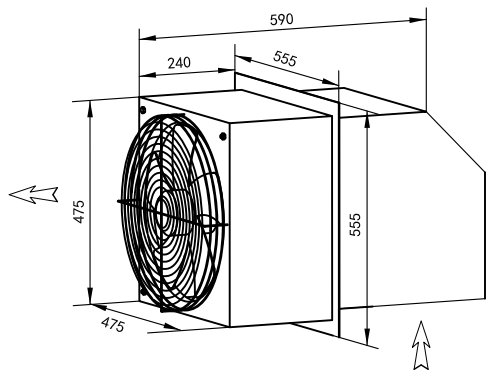
边墙送风机 WEXR-S400
