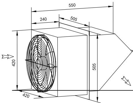
边墙排风机 WEXR-P350
