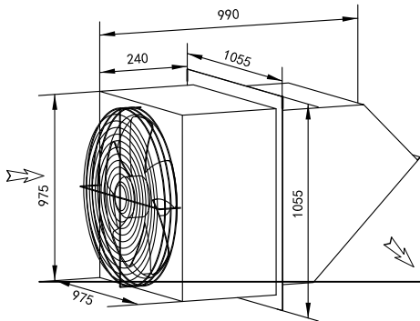
边墙排风机 WEXR-P750
