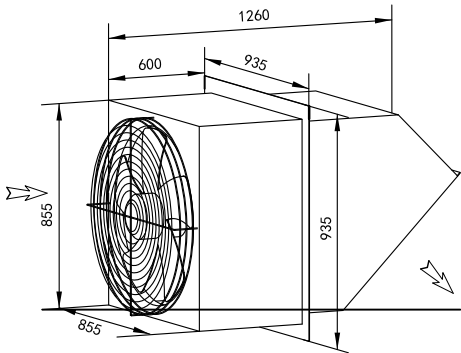
边墙排风机 WEXR-PL700
