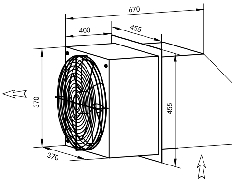
边墙送风机 WEXR-SL300
