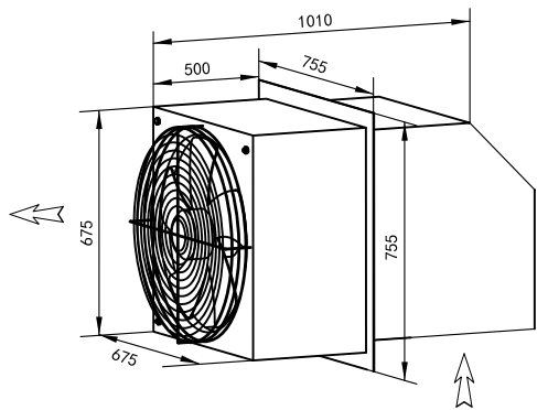
边墙送风机 WEXR-SL600
