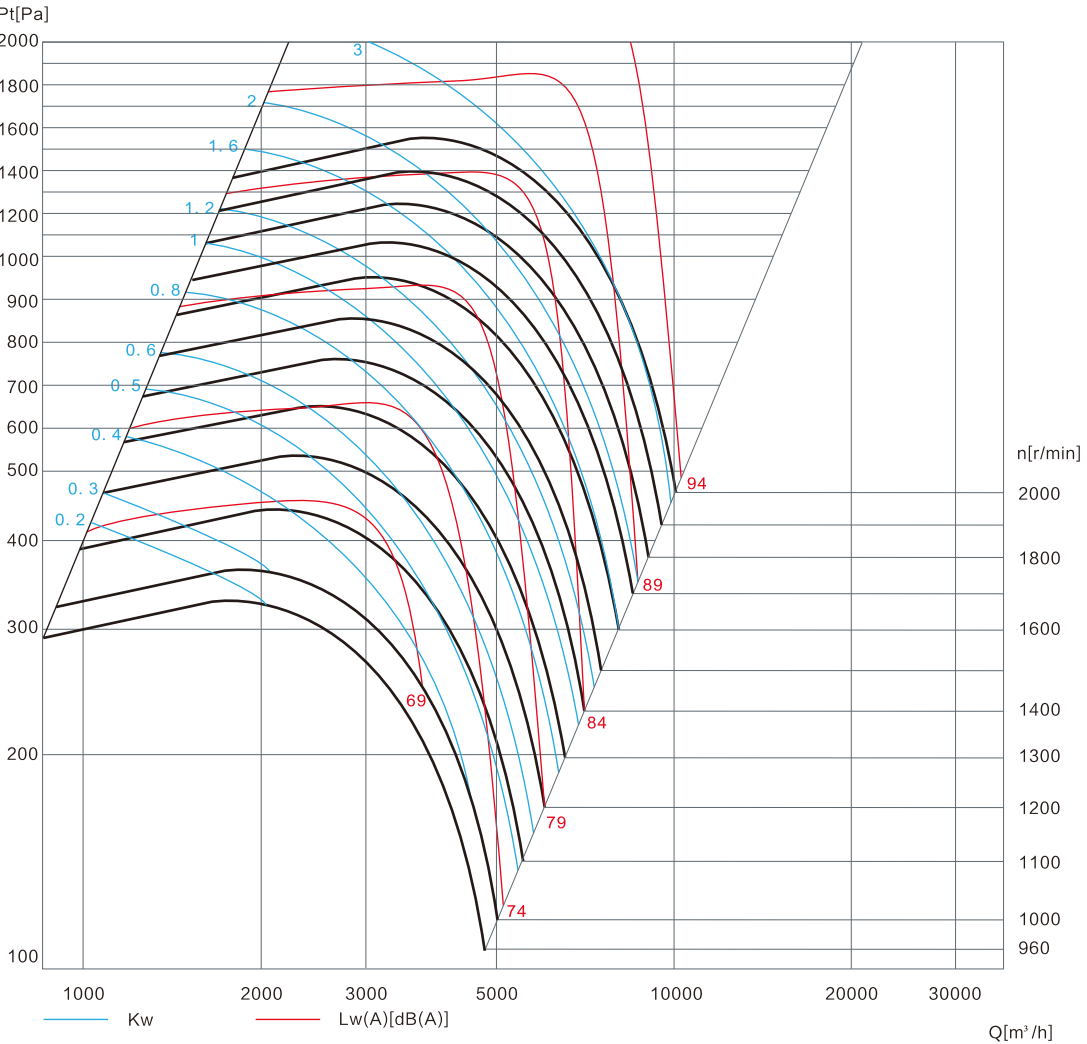
RHA 450 无蜗壳风机箱 RHA 450 No scroll fan case
