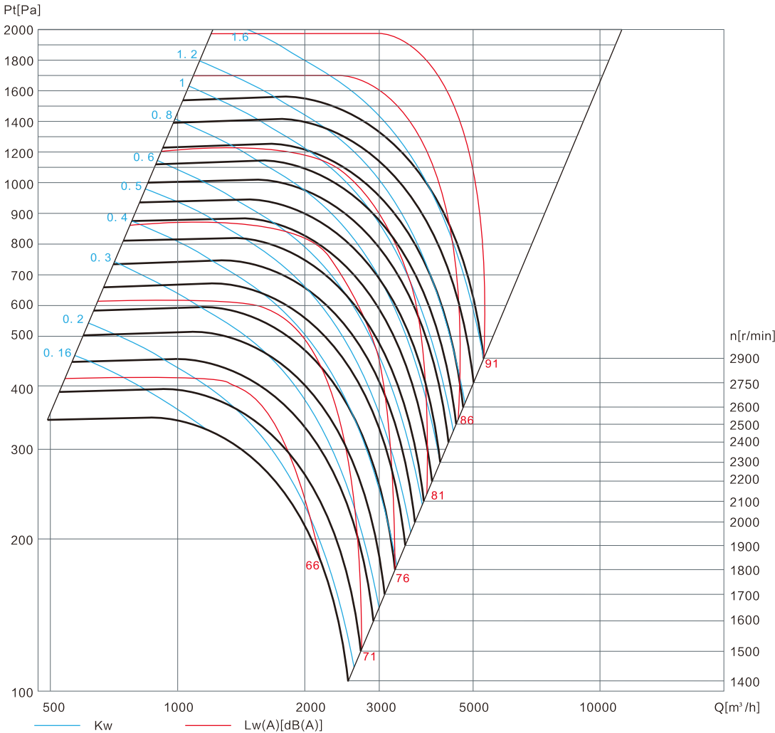
RHA 315 无蜗壳风机箱 RHA 315 No scroll fan case
