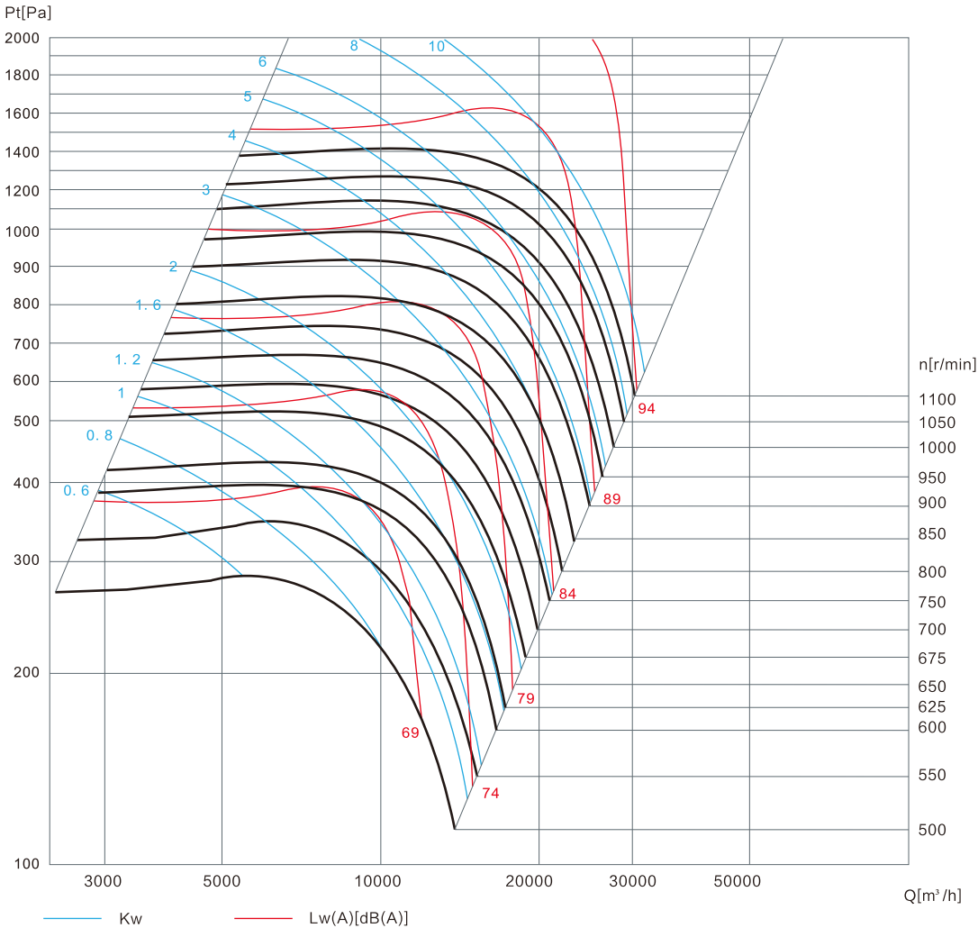
RHA 800 无蜗壳风机箱 RHA 800 No scroll fan case
