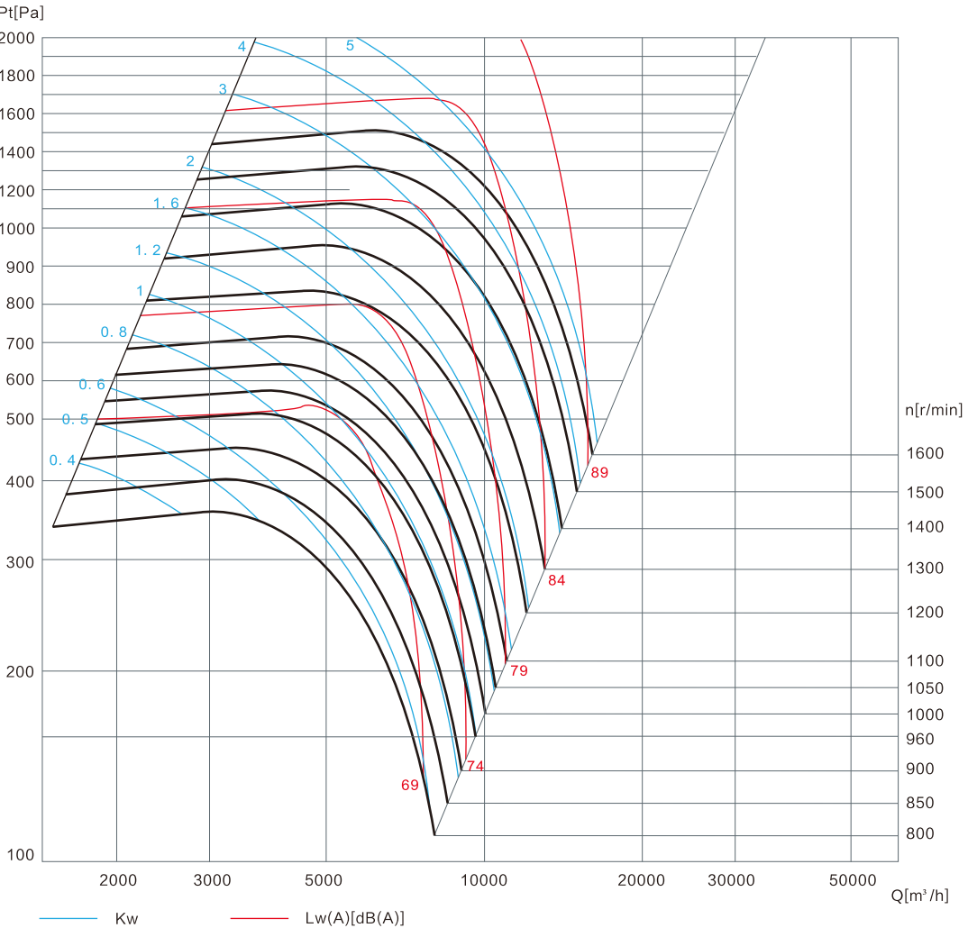
RHA 560 无蜗壳风机箱 RHA 560 No scroll fan case
