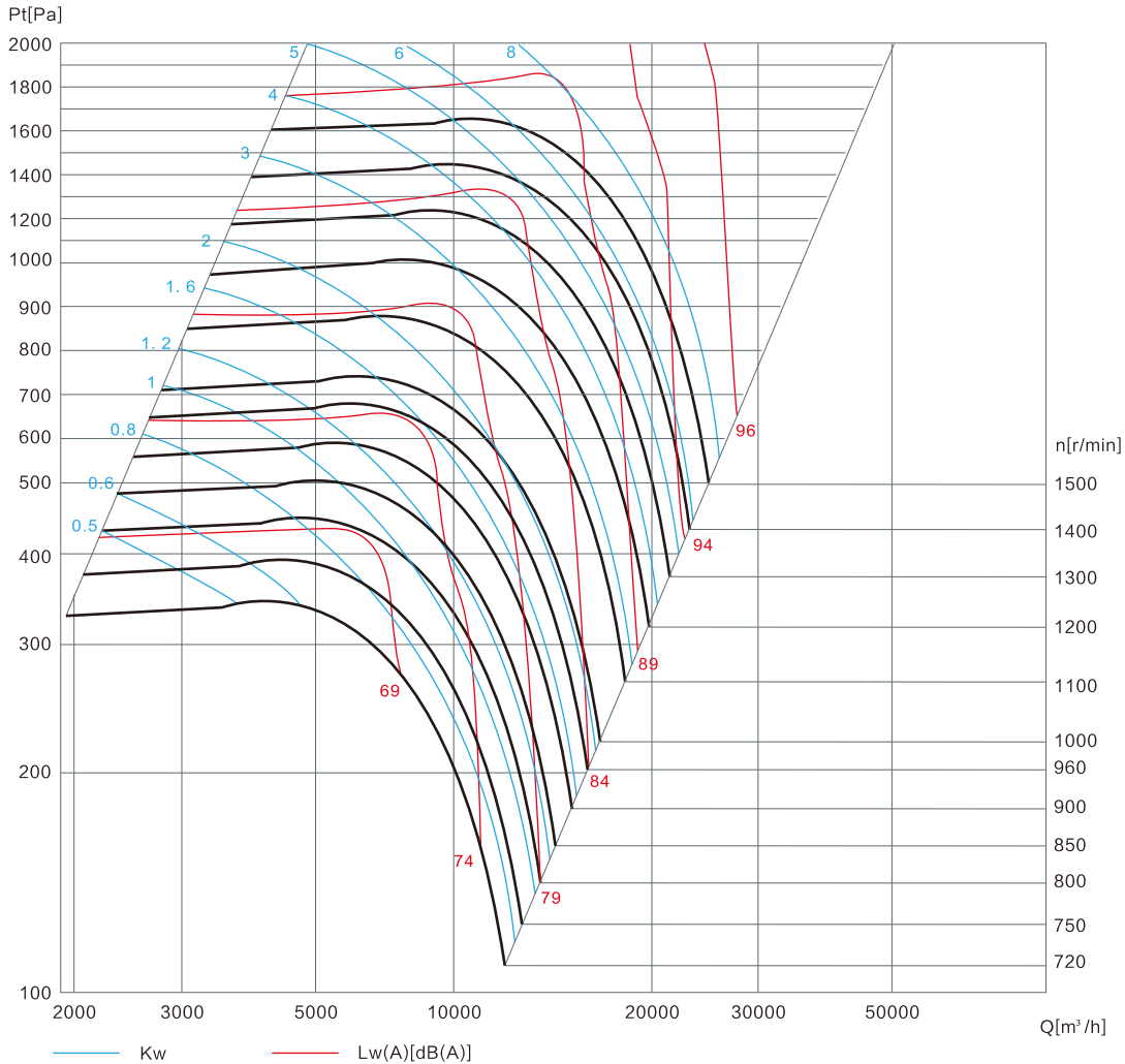
RHA 630 无蜗壳风机箱 RHA 630 No scroll fan case
