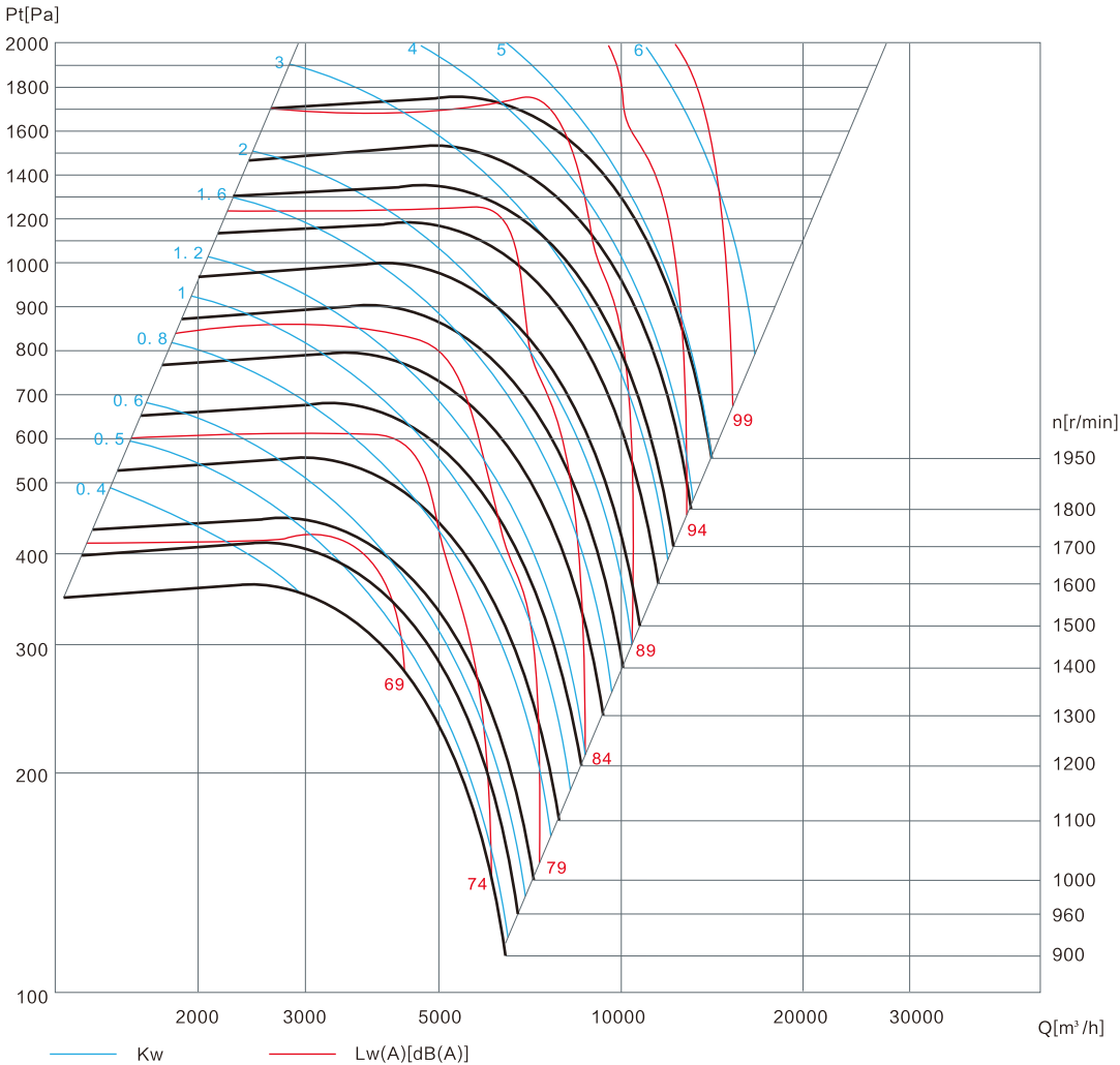
RHA 500 无蜗壳风机箱 RHA 500 No scroll fan case
