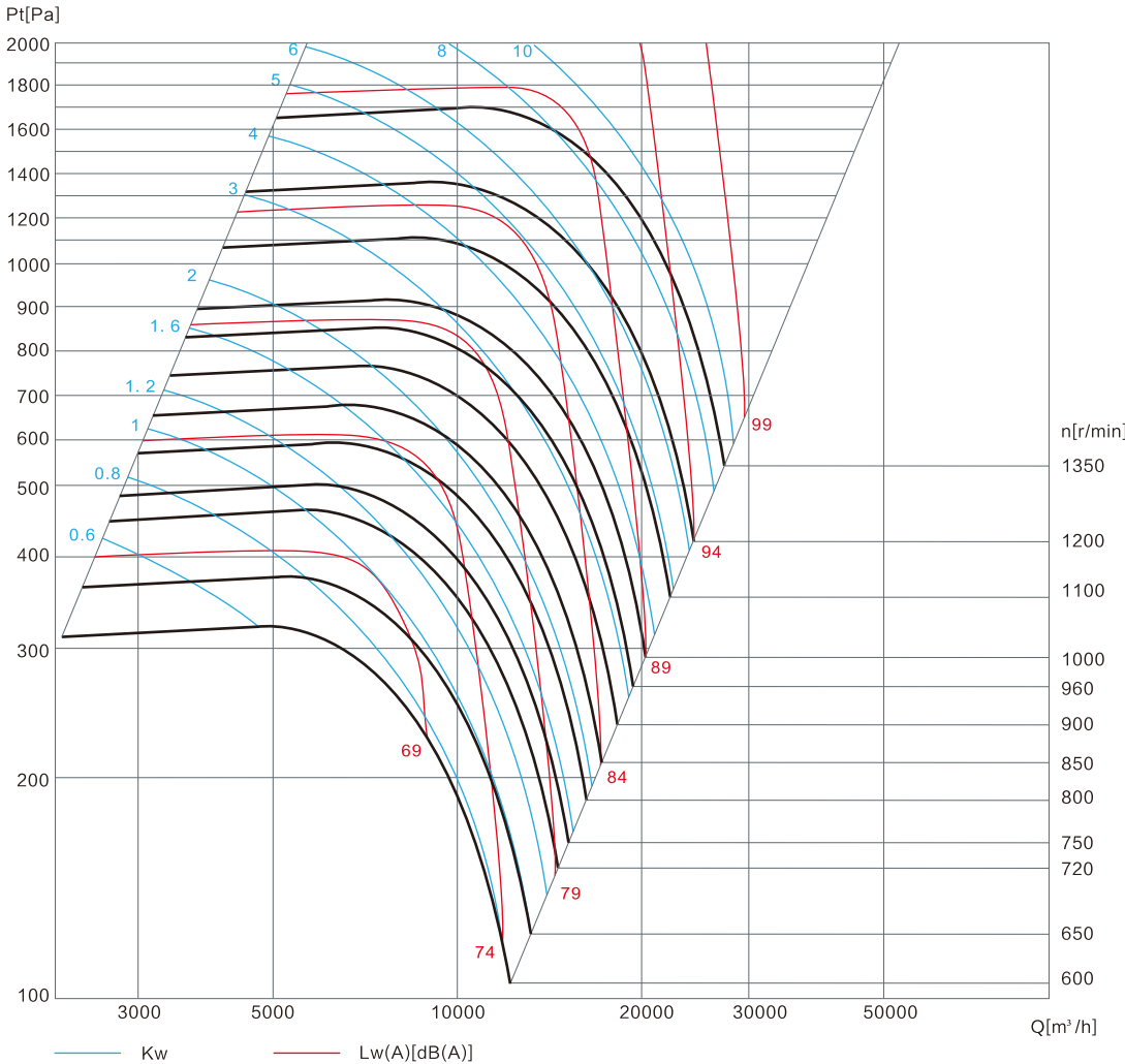
RHA 710 无蜗壳风机箱 RHA 710 No scroll fan case
