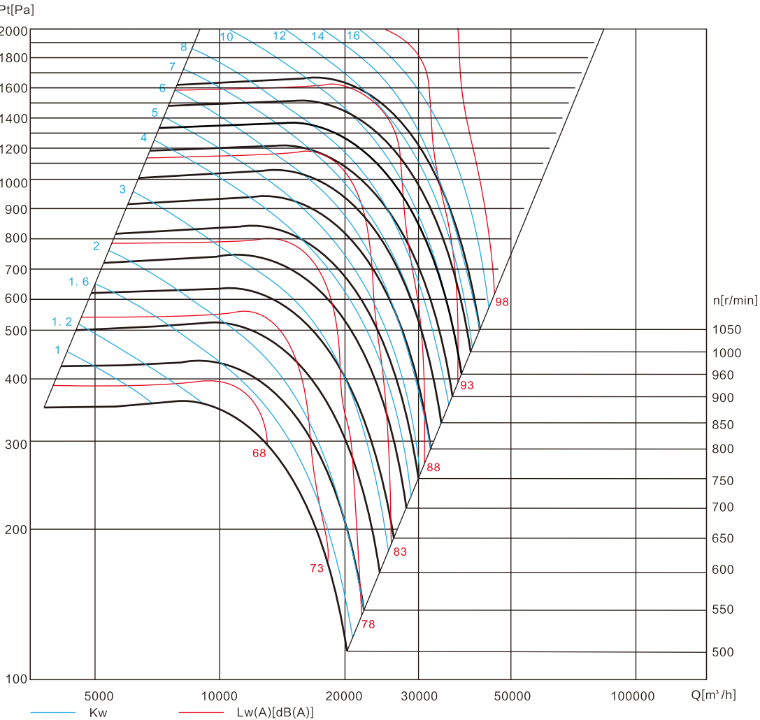
RHA 900 无蜗壳风机箱 RHA 900 No scroll fan case
