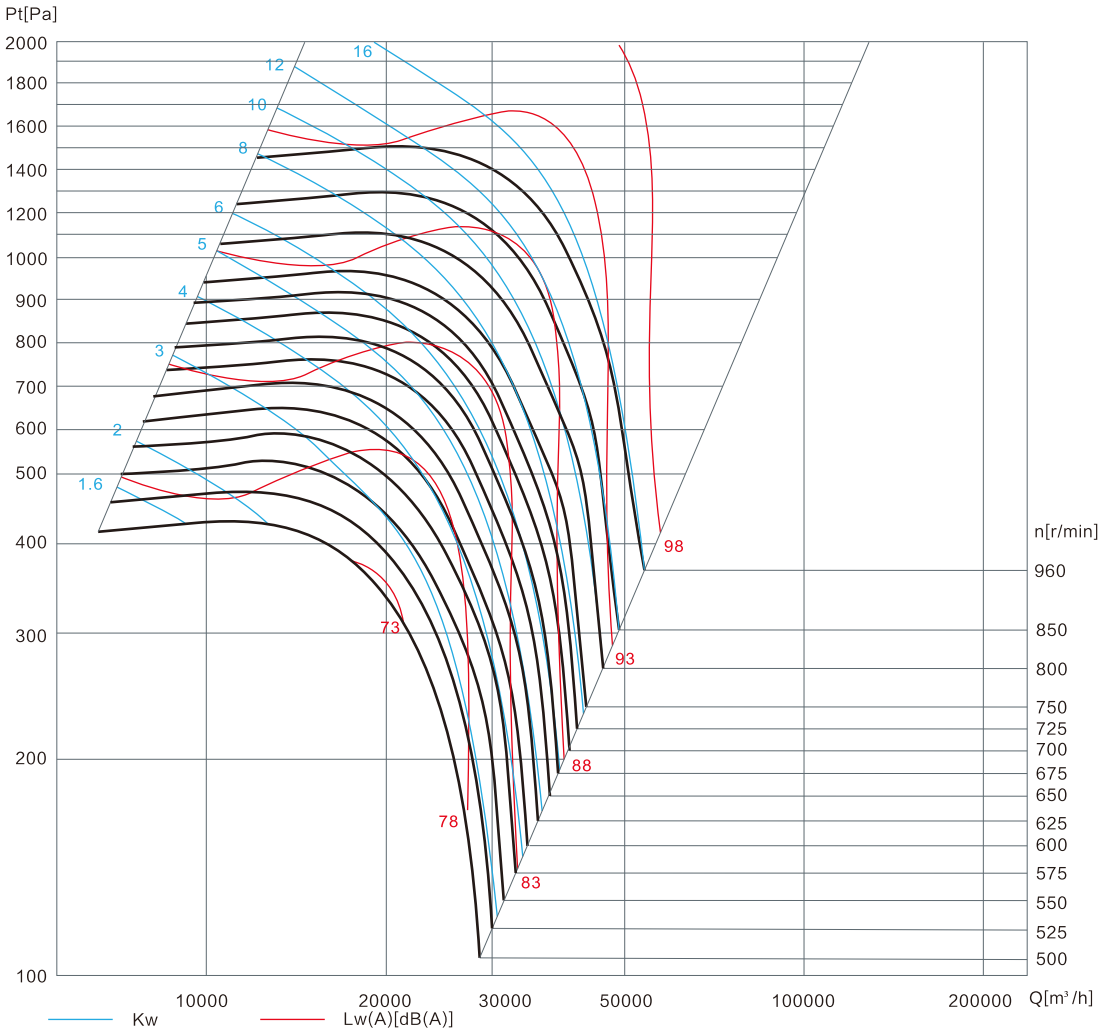
RHA 1000 无蜗壳风机箱 RHA 1000 No scroll fan case
