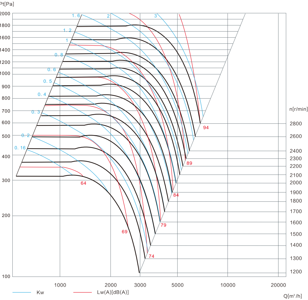
RHA 355 无蜗壳风机箱 RHA 355 No scroll fan case
