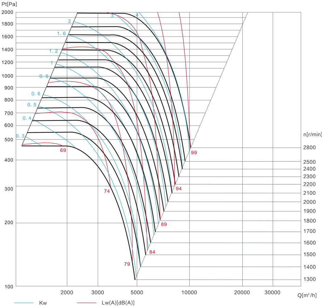
RHA 400 无蜗壳风机箱 RHA 400 No scroll fan case
