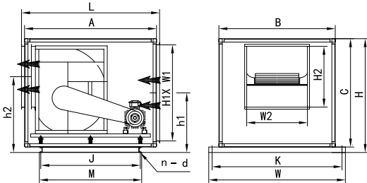
电机内置左 水平进风水平顶出 （MIL H0HT）
