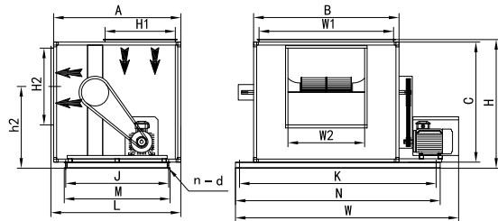
电机侧置左 垂直顶进水平顶出 (MSL VTHT)
