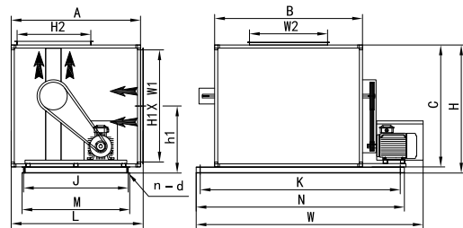
电机侧置左 水平进风垂直顶出 (MSL H0VT)
