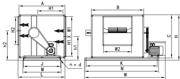
电机侧置左 水平进风水平顶出 （MSL H0HT）
