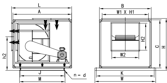
电机内置左 垂直顶进水平顶出 （MIL VTHT）
