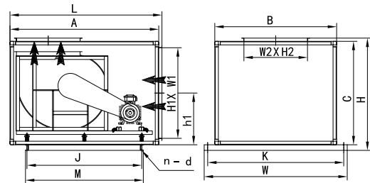
电机内置左 水平进风垂直顶出 （MIL H0VT）
