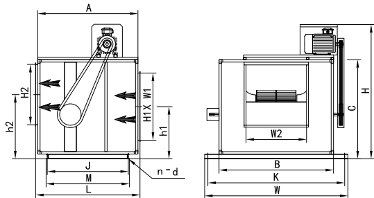
电机顶置左 水平进风水平顶出 （MTL H0HT）
