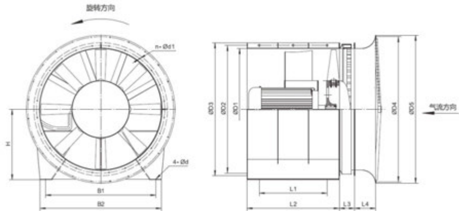
单向轴流风机几何尺寸（卧式）
